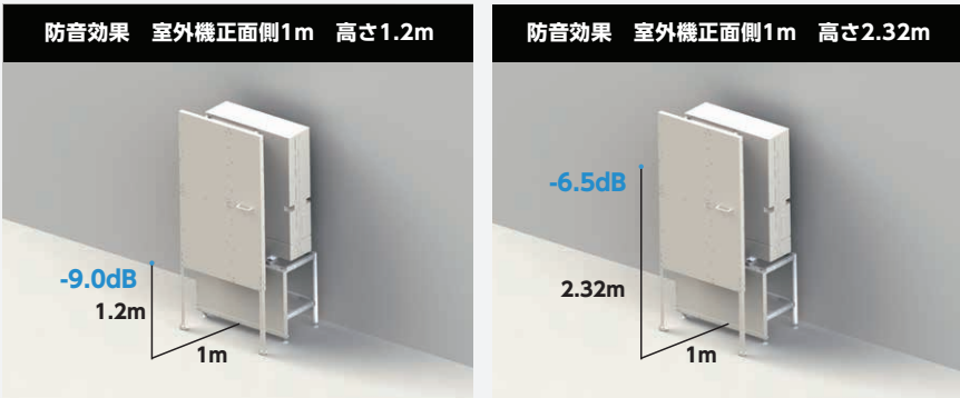
正面側1m 高さ2.32m地点での防音効果周波数特性値
