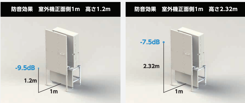
正面側1m 高さ2.32m地点での防音効果周波数特性値
