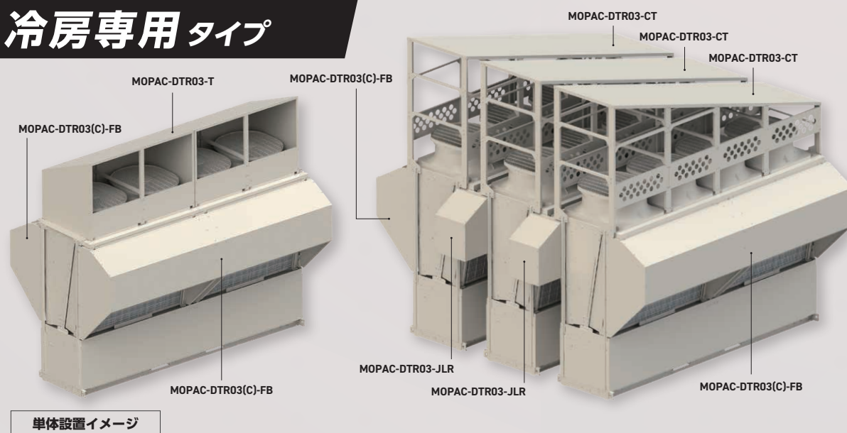
連結設置イメージ( 室外機 3 台 )
