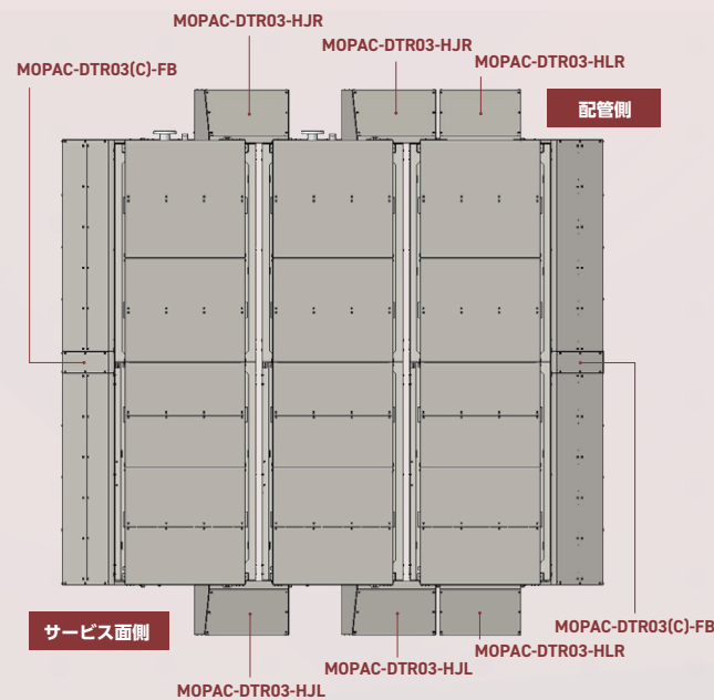
連結設置時（室外機 3 台） 吸込側構成図
