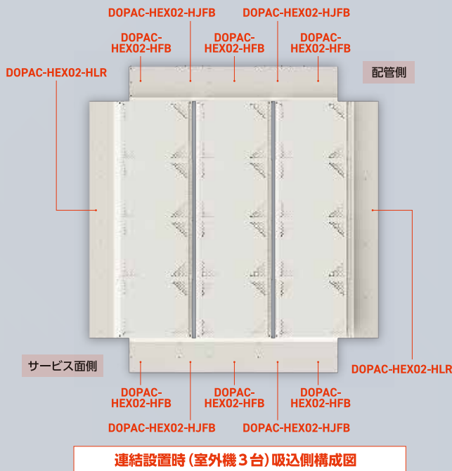
連結設置時(室外機3台)吸込側構成図
