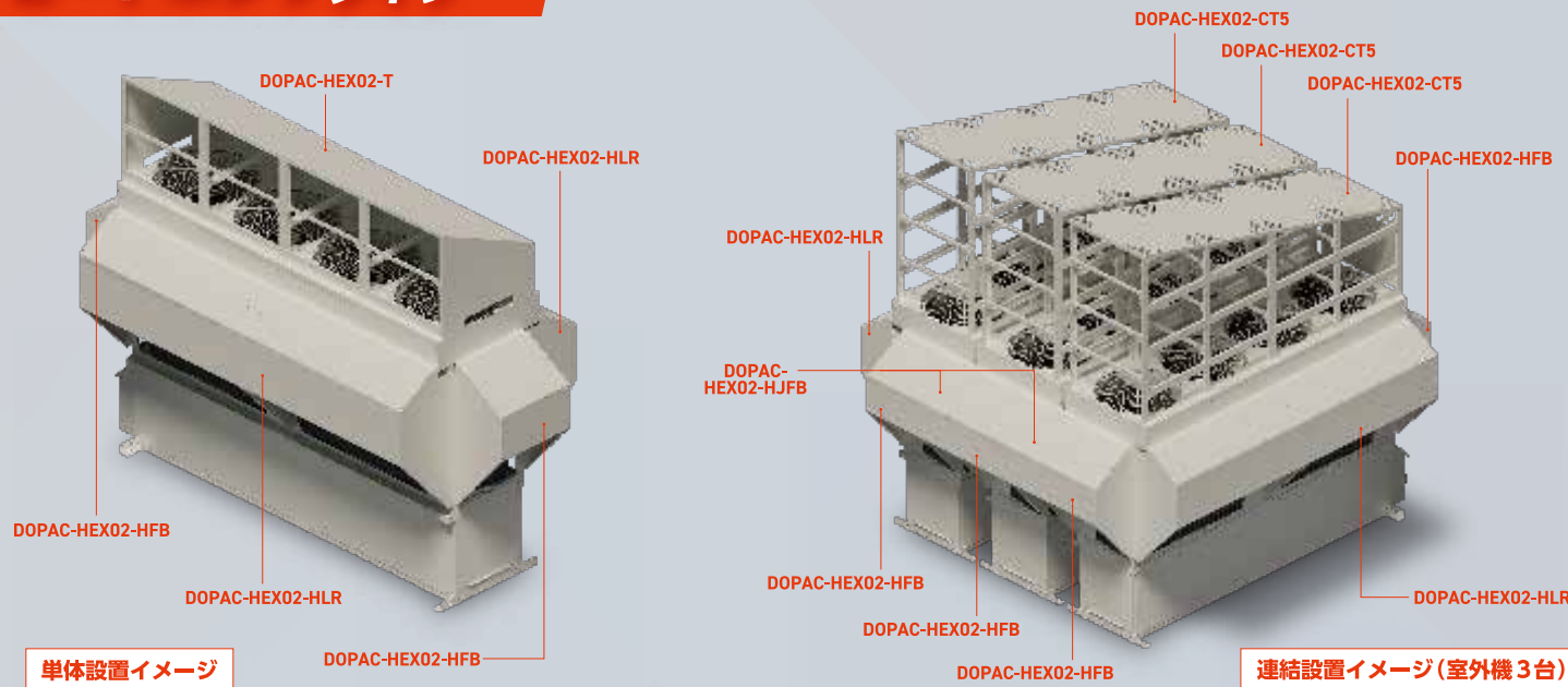
単体設置イメージ
