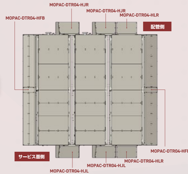
連結設置時 (室外機 3台) 吸込側構成図
