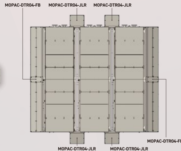
連結設置時 (室外機 3台) 吸込側構成図
