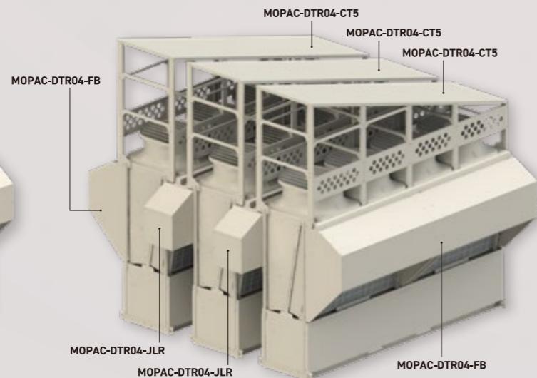
連結設置イメージ (室外機 3台)
