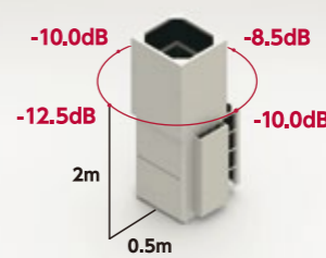
防音効果 室外機周囲0.5m 高さ2m
