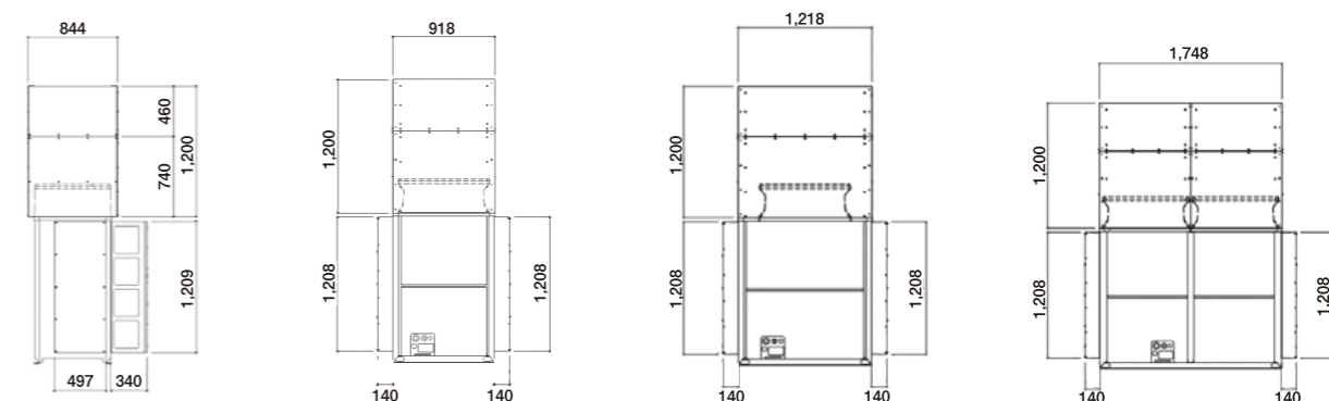
側面図(各型名共通) MOSGD-B01-ST-(ZM/K/BSG/S) MOSGD-B02-ST-(ZM/K/BSG/S) MOSGD-B03-ST-(ZM/K/BSG/S)
