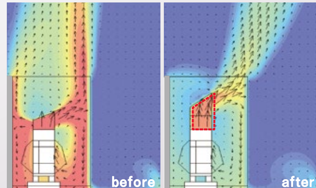
▶気流解析コンター図
